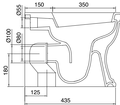
SEZIONE A-A
