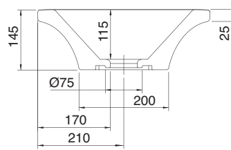
SEZIONE A-A
